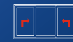
3-teiliges Element mit 2 Hebe-Schiebeflügeln und Festverglasung
